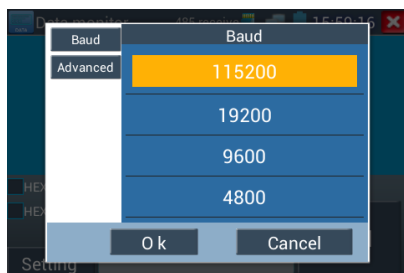
Рис.3.3.14-1 Настройка мониторинга данных по протоколу RS485
