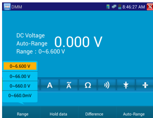
Рис.3.3.17-2 Выбор режима измерений
