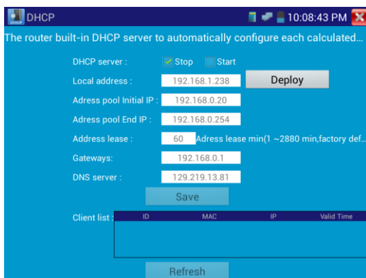
Рис.3.3.27-7 Настройка DHCP-сервера
