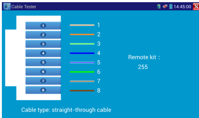
Рис. 3.3.11-1 Тестер кабеля
