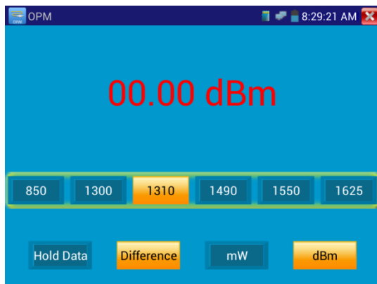
Рис. 3.3.15-2 Измерение относительной оптической мощности
